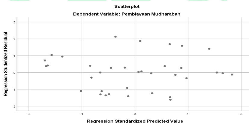
Gambar 4.1 scatteplot
